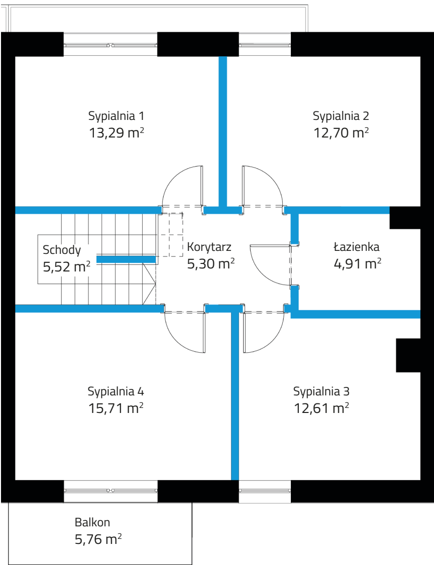
Piętro 70,04 m 2
