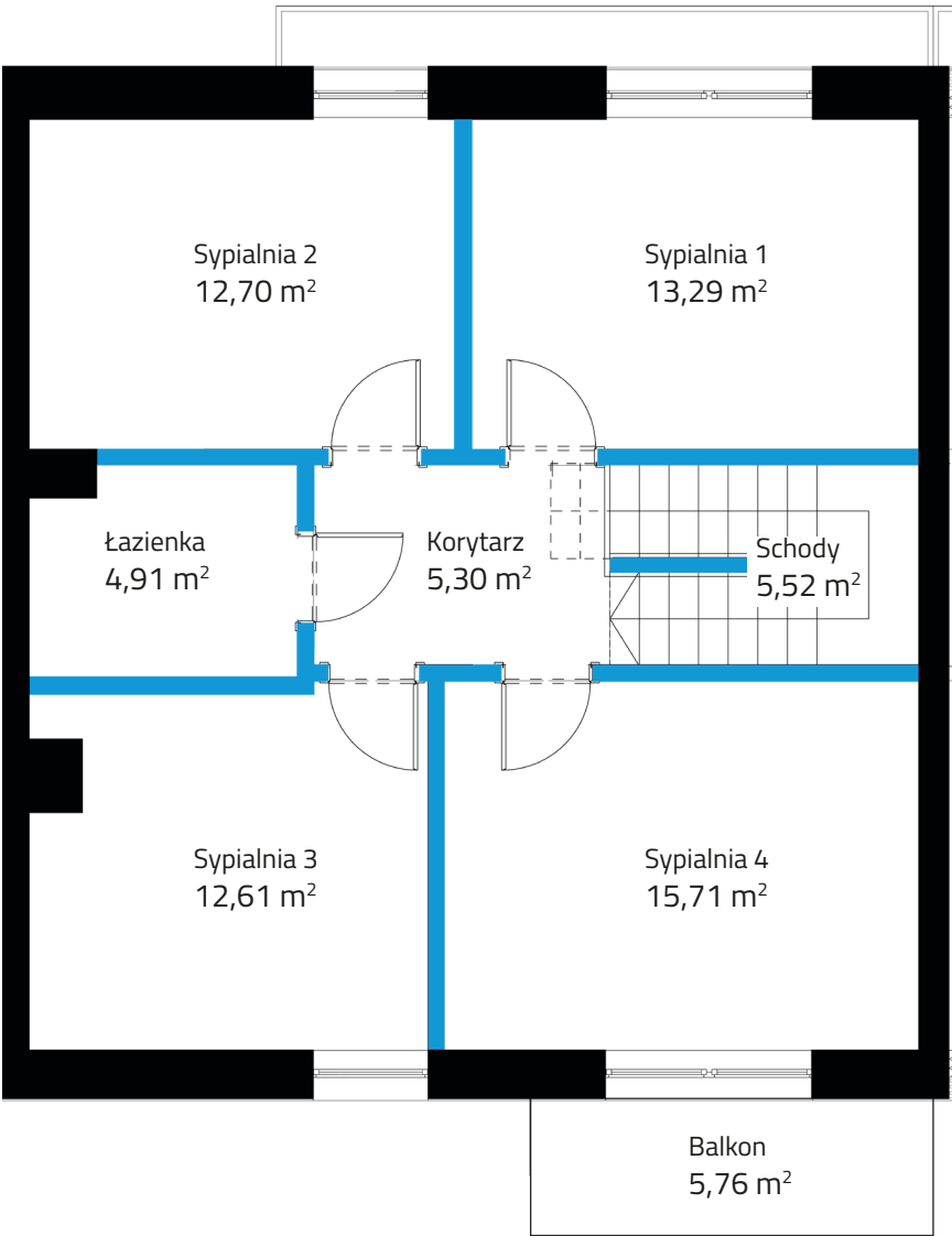
Piętro 70,04 m 2
