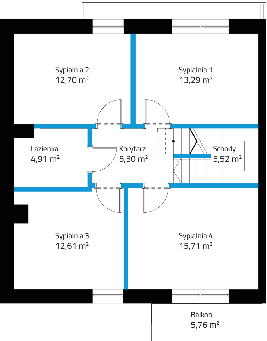
Piętro 70,04 m 2
